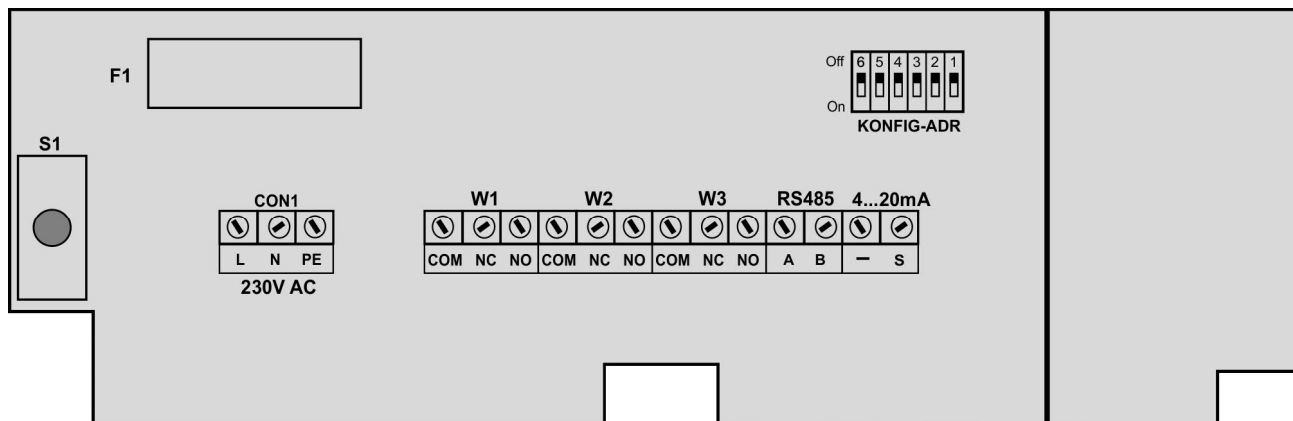
Rys.2. Listwa zaciskowa
