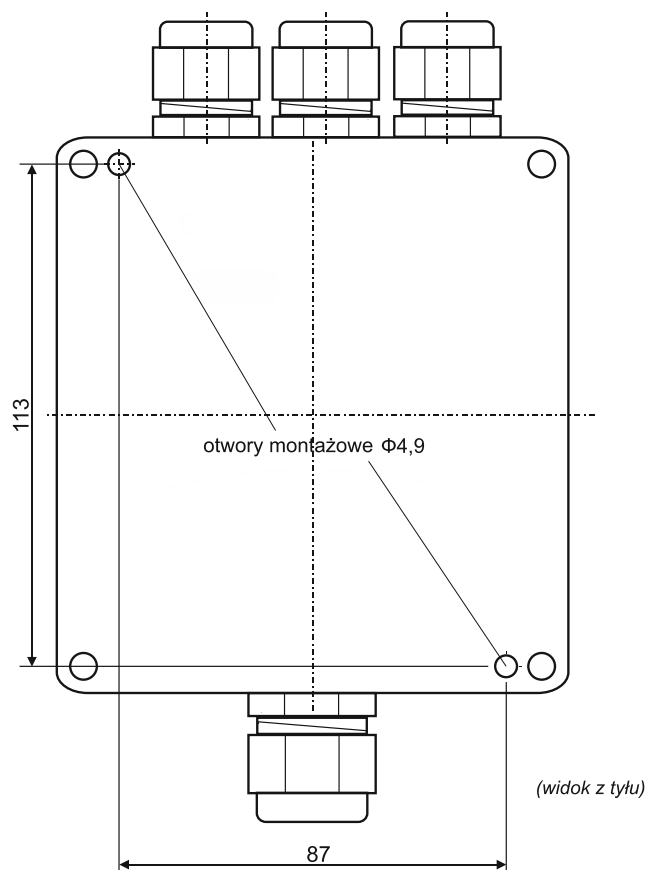
Rys.3. . Tmaster CO/LPG/NO2 L/EPE/D – moduł główny (CO) - wymiary
