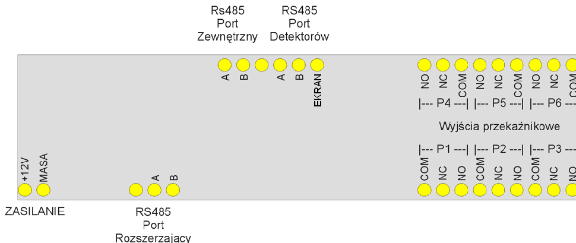
Rys. 1. – Opis zacisków kontrolera detekcji gazów DINster®3xRS
